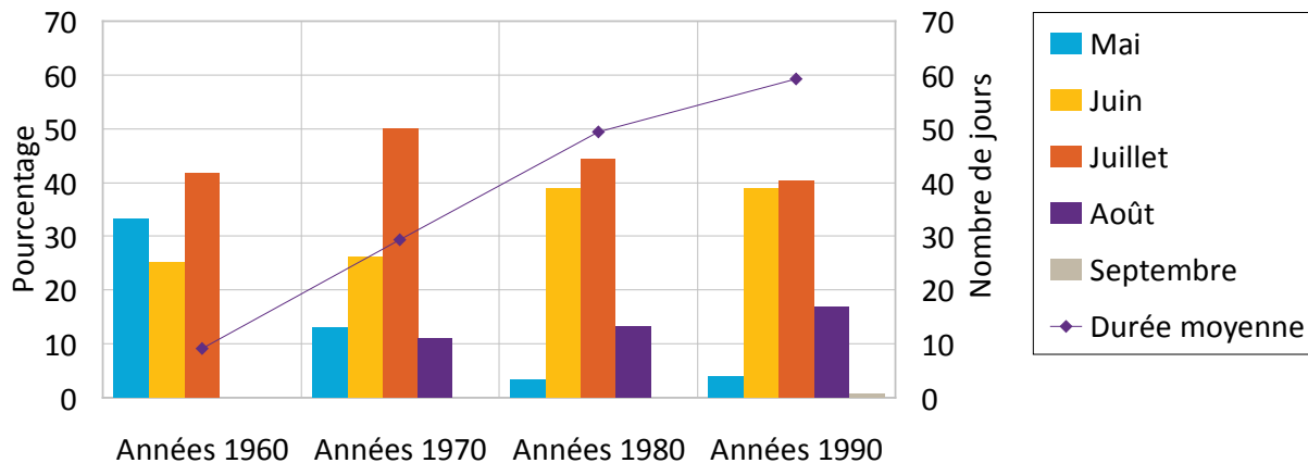
Figure 21. Proportion des grands incendies qui se produisent chaque mois dans l'écozone + des plaines hudsoniennes et durée moyenne de la saison active des feux (ligne mauve), des années 1960 aux années 1990.
