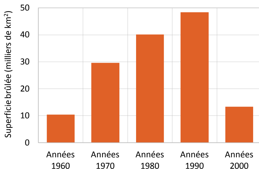
Figure 14. Total de la superficie brûlée par les grands incendies dans l'écozone + de la taïga des plaines, par décennie, des années 1960 aux années 2000.
